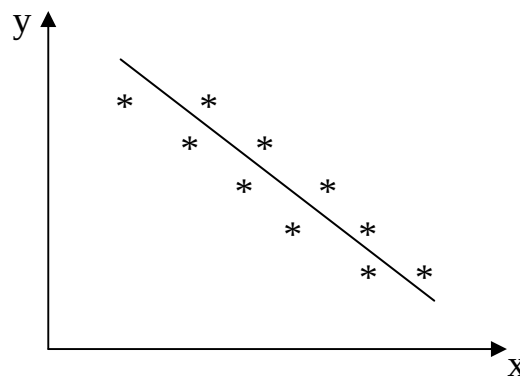
Dépendance linéaire forte.
