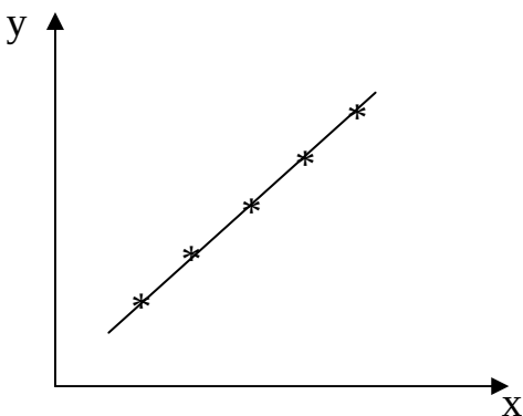
Dépendance linéaire parfaite.
